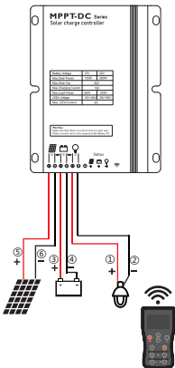
图1、2.4G遥控通信
