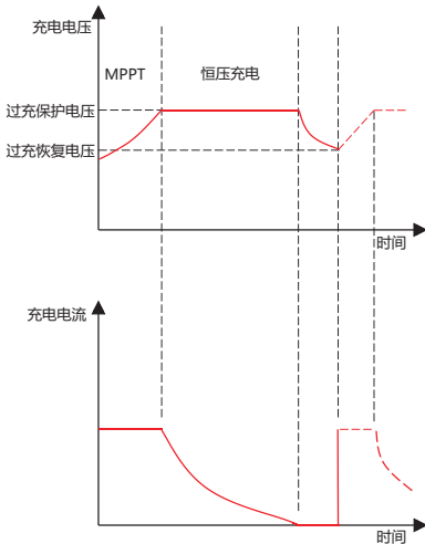
图2-3 锂电池充电曲线
