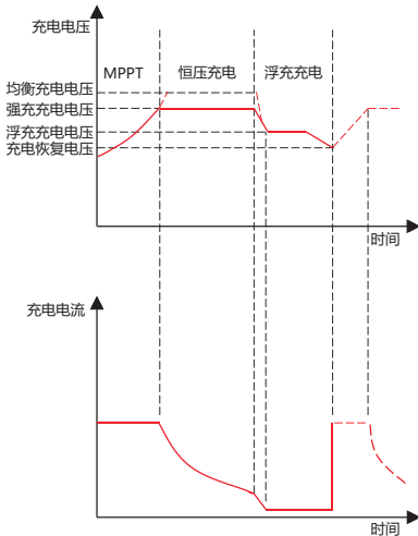
图2-2 铅酸电池充电曲线
