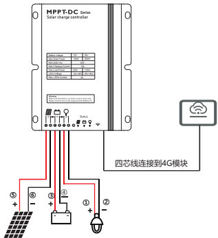
图3、4G物联网模块通信
